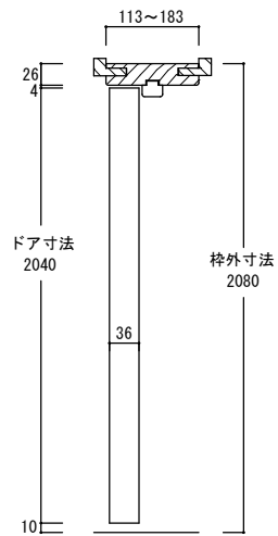
縦断面図
