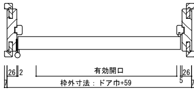
横断面図
