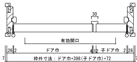
横断面図・親子
