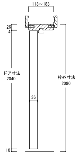
縦断面図
