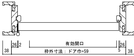
横断面図・親子
