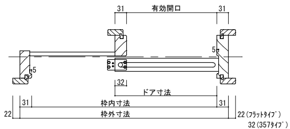
引違い 横断面図
