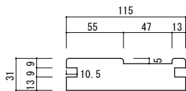
縦枠
