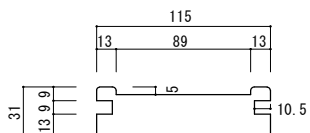
縦枠
