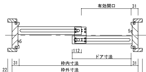
引違い 横断面図
