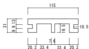
上枠
