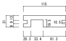
上枠
