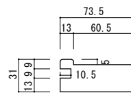
戸当り
