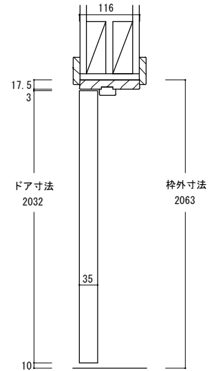
縦断面図
