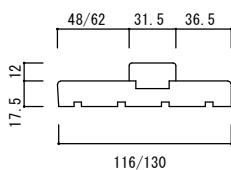
内部用ドア枠
