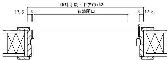
シングルドア 横断面図
