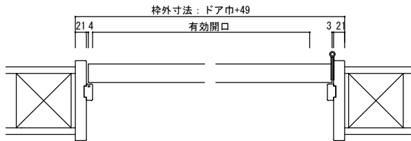
横断面図
