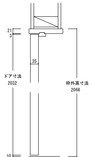
縦断面図
