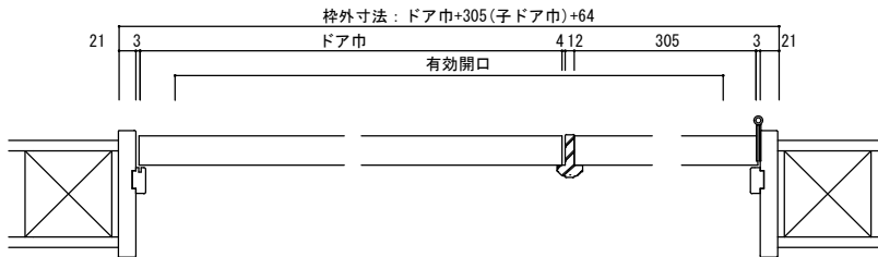
横断面図
