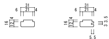
戸当り
