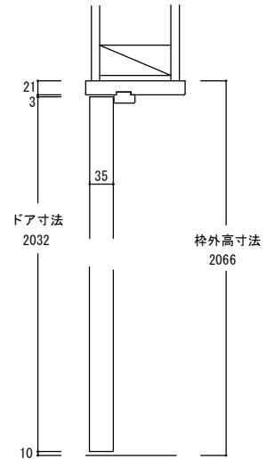
縦断面図
