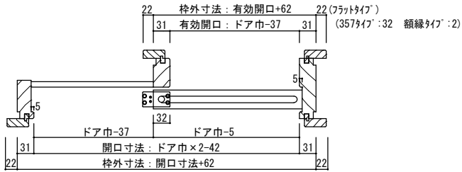
片引き 横断面図
