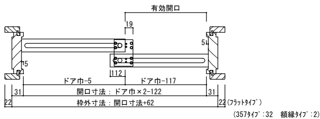
引違い 横断面図
