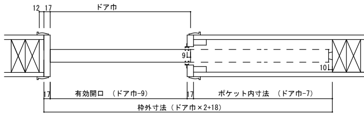
横断面図
