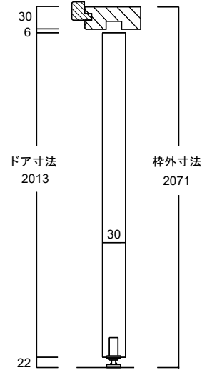
縦断面図
