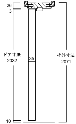
縦断面図
