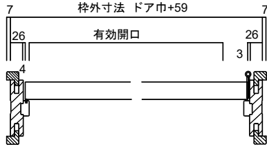
横断面図
