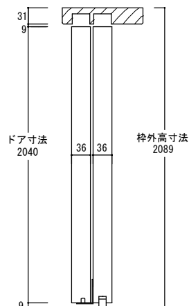
縦断面図
