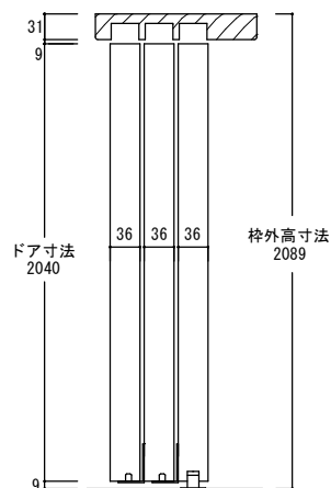
縦断面図
