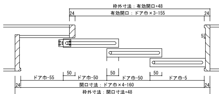
横断面図
