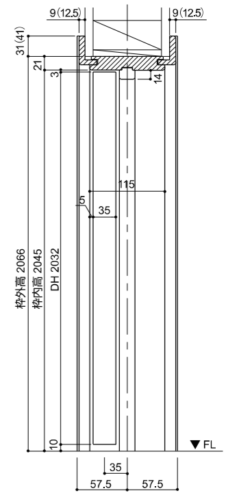
縦断面図
