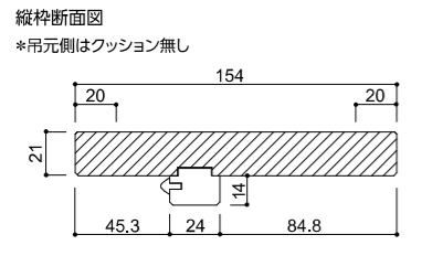
固定枠断面図
