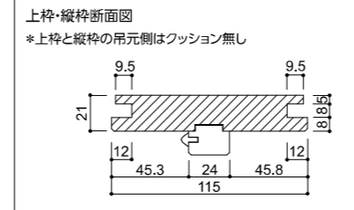
差込枠断面図
