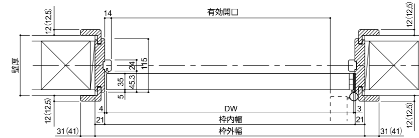
横断面図
