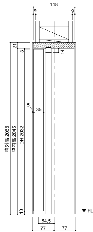
縦断面図
