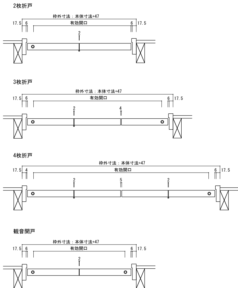
横断面図
