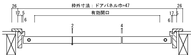
3枚折戸
