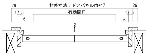
観音開戸
