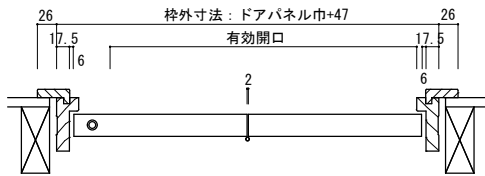
2枚折戸
