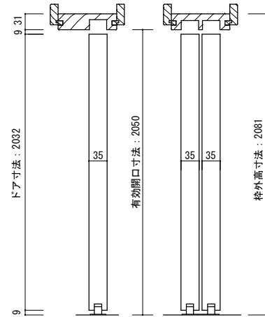
片引き 引違い
