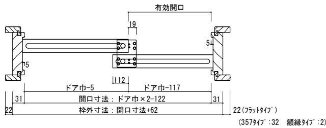
引違い 横断面図
