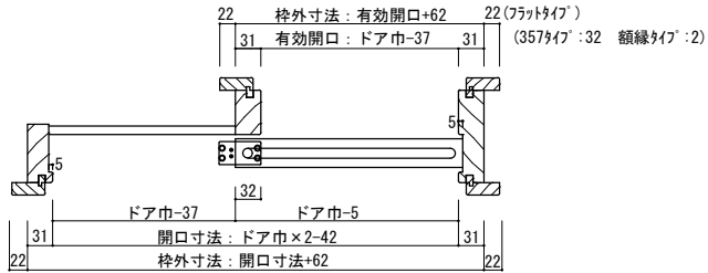
片引き 横断面図
