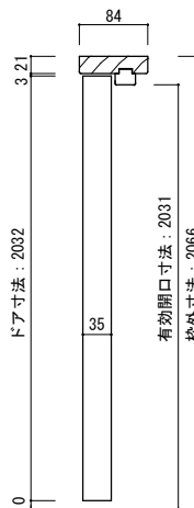
縦断面図
