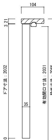
縦断面図
