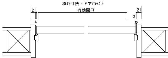
横断面図
