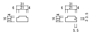
戸当り
