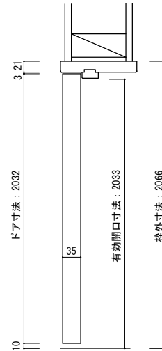
縦断面図
