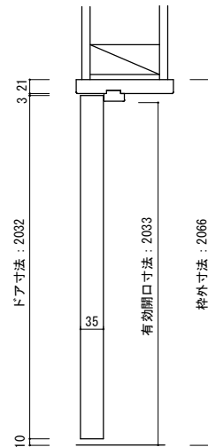
縦断面図
