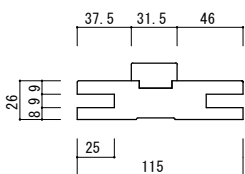
内部ドア枠（差込型）
