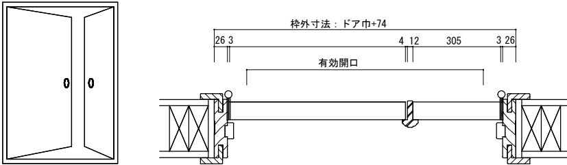
親子ドア 横断面図
