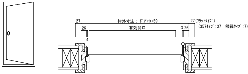
シングルドア 横断面図
